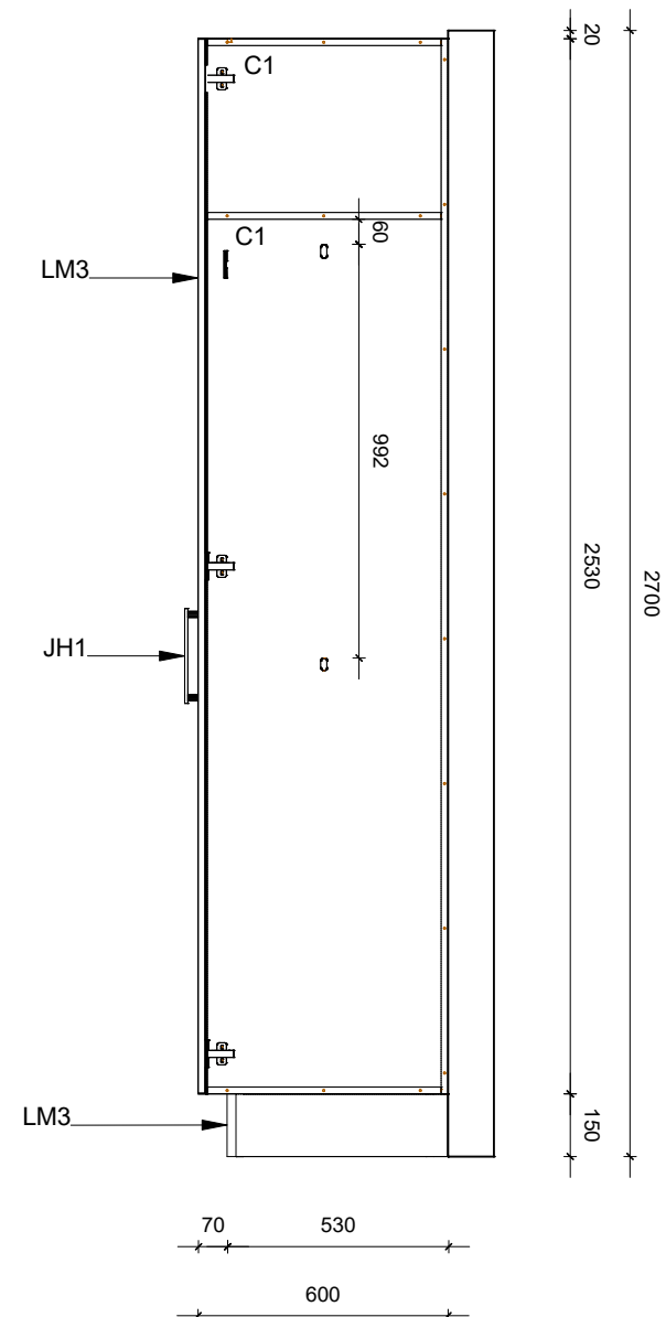
Section B Scale: 1 : 20
