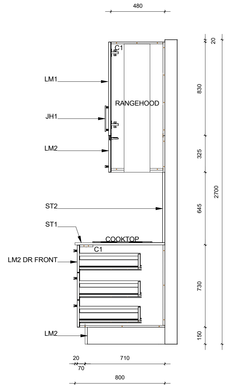
Section C Scale: 1 : 20
