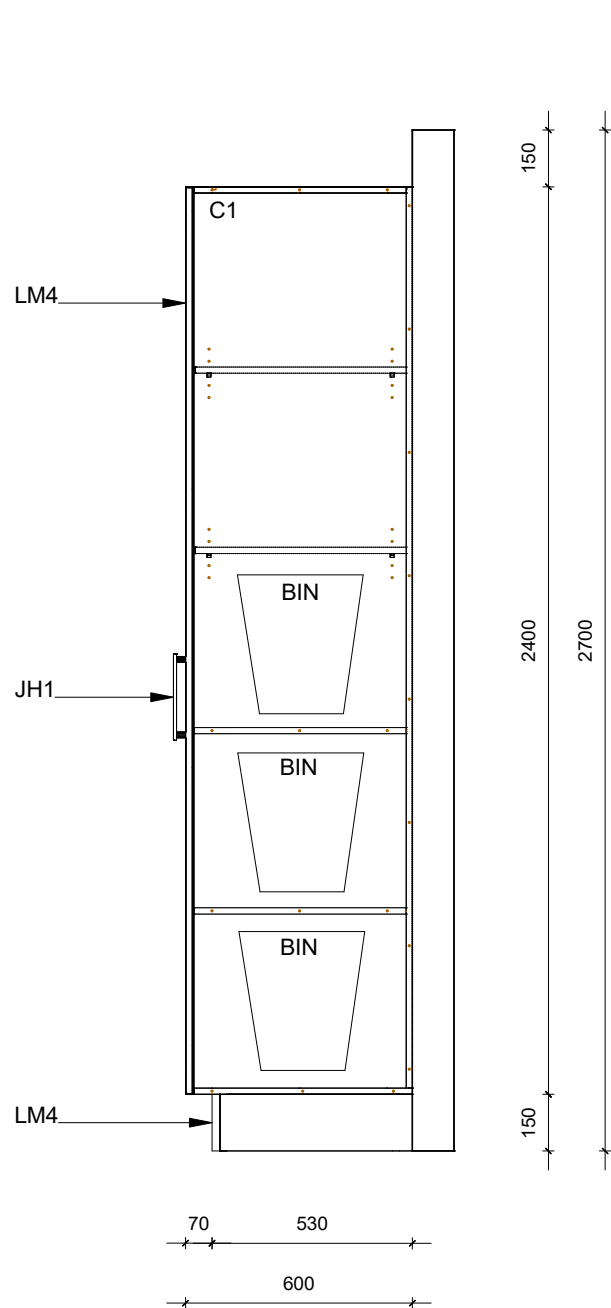
Section A Scale: 1 : 20
