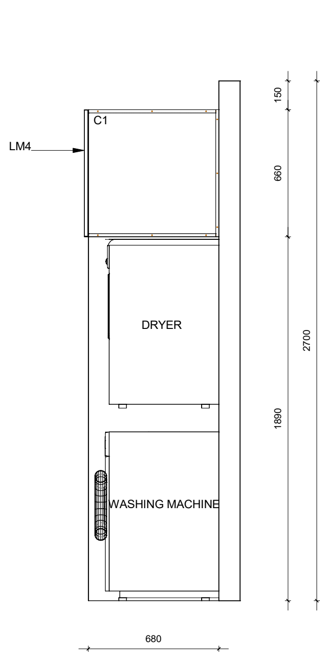
Section D Scale: 1 : 20
