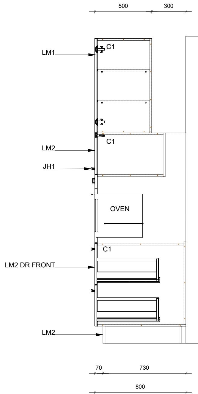
Section A Scale: 1 : 20
